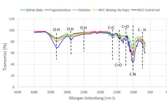
Gambar 3. Grafik spektrum FTIR bahan baku, lignoselulosa, selulosa dan MCC batang ubi kayu
