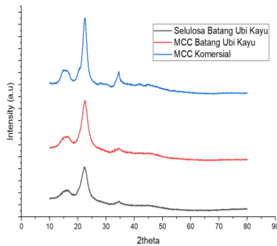
Gambar 7. Difraksi XRD pada masing-masing sampel.
